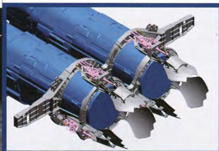
Uno schema del sistema TVC applicato ai propulsori dell'X-2.
