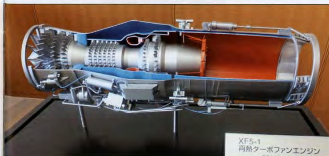
Uno spaccato del motore XF5-1, sviluppato dalla giapponese IHI.
